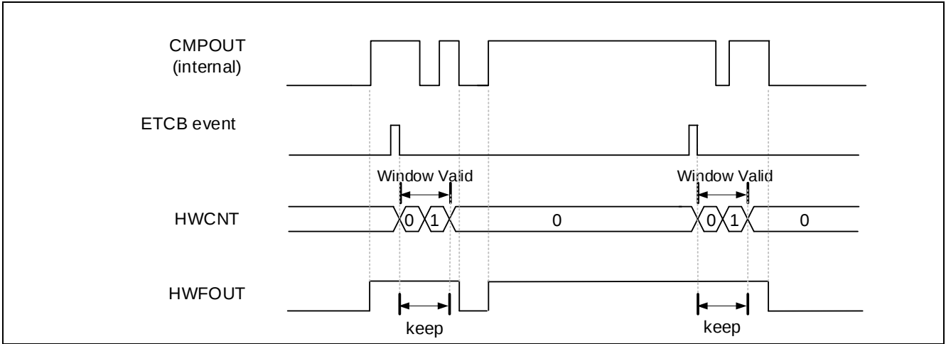
Figure 10-3 硬件窗口滤波机制
