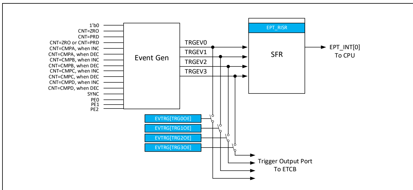
Figure 14-38 同步触发输出
