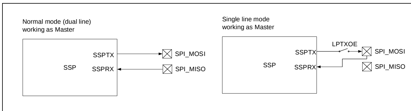
Figure 16-2 SPI 单线通讯模式
