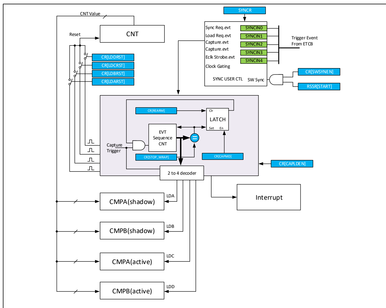
Figure 13-12 捕捉模式结构框图
