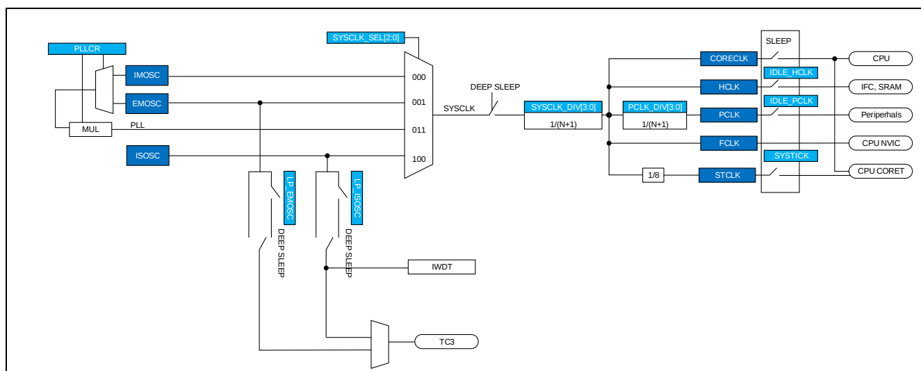
Figure 5-1 时钟结构示意图
