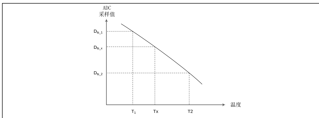
Figure 9-10 ADC采样内部温度传感器
