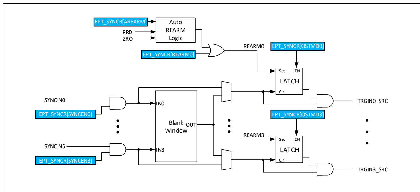
Figure 14-37 同步触发输入
