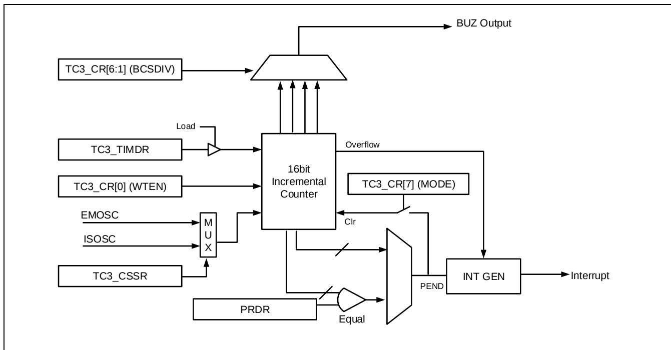
Figure 12-1 时钟定时器模块框图
