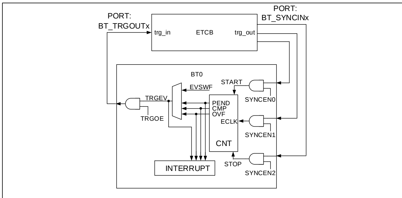
Figure 11-4 同步触发原理
