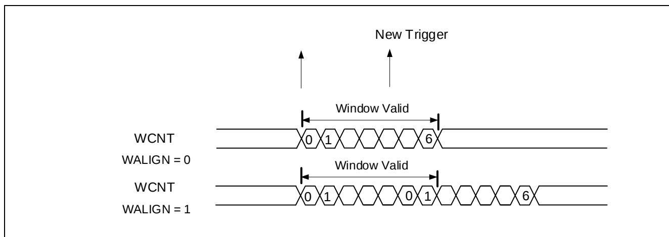
Figure 10-5 SWFCR[WALIGN]不同值时，窗口和触发信号的关系
