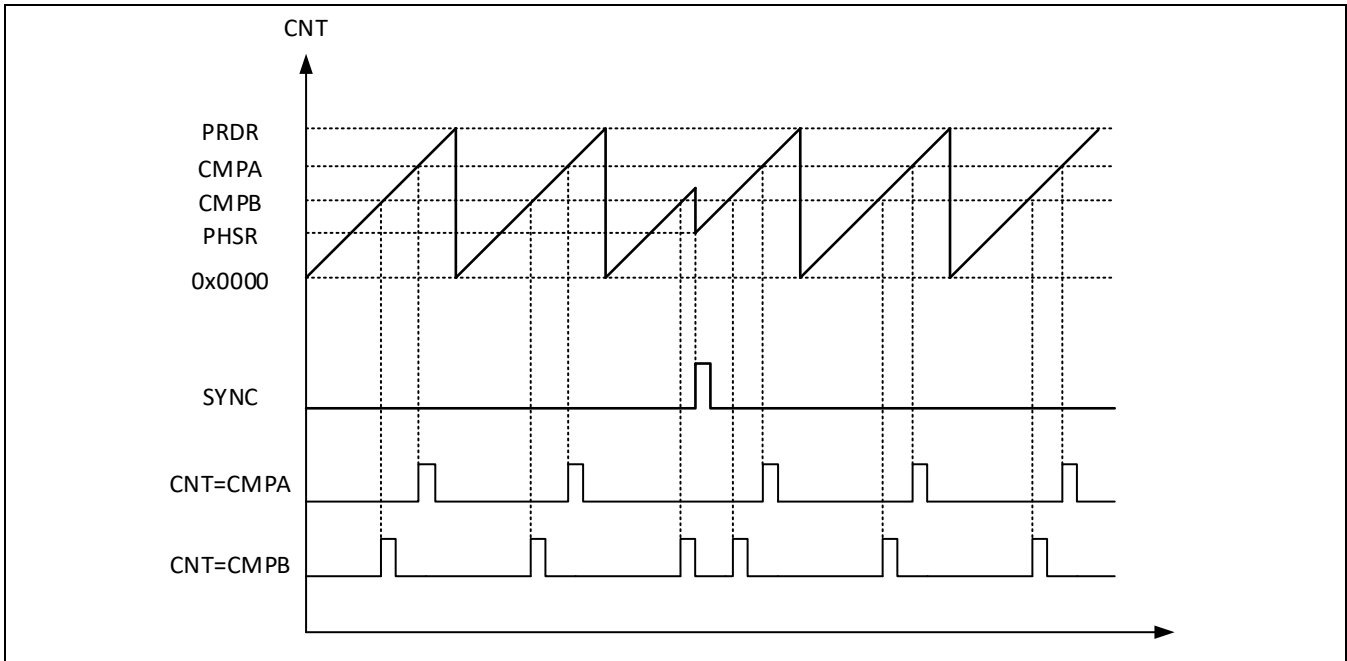
Figure 13-9 递增模式下比较事件产生时序
