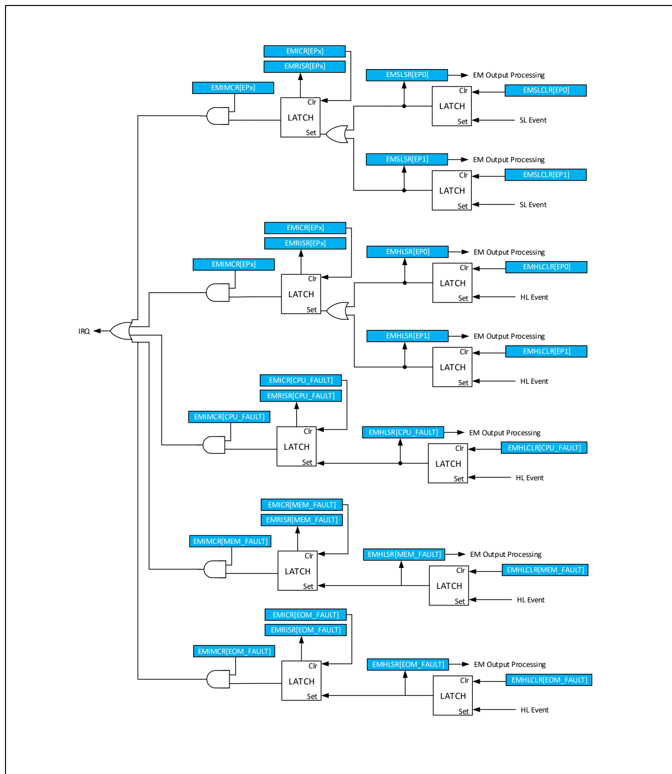
Figure 14-34 紧急模式中断
