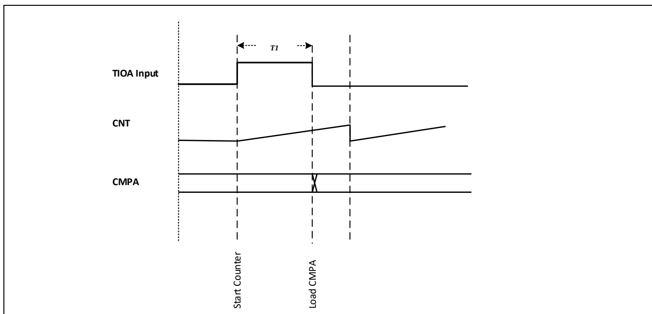
Figure 13-14 测量TIOA的脉冲宽度
