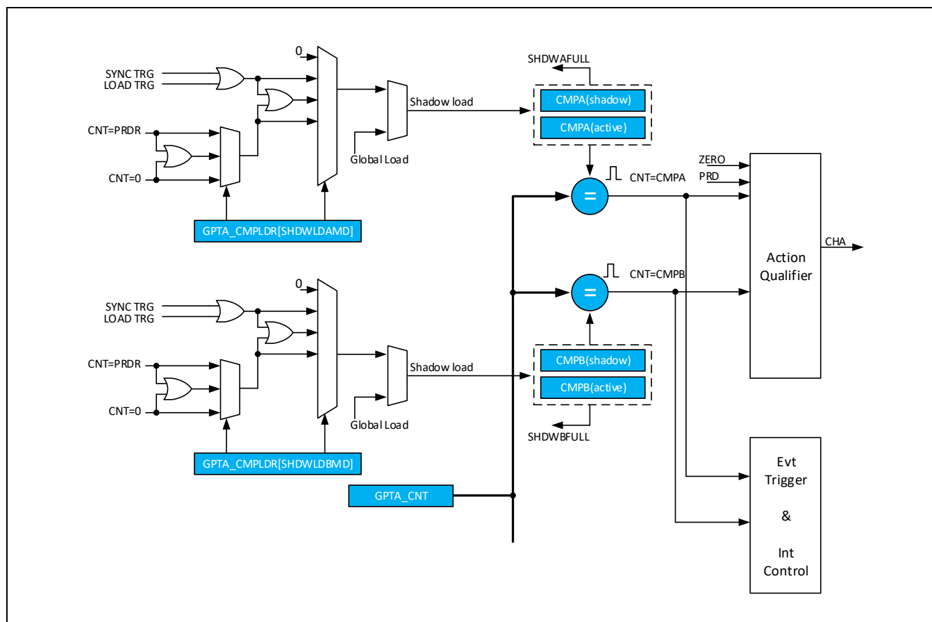
Figure 13-8 计数器值比较控制
