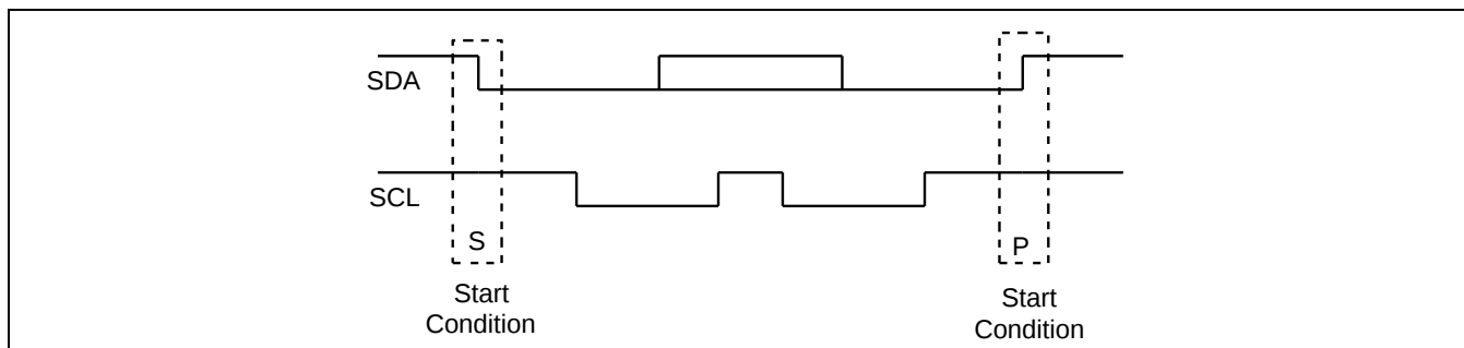
Figure 17-3 起始位和停止位
