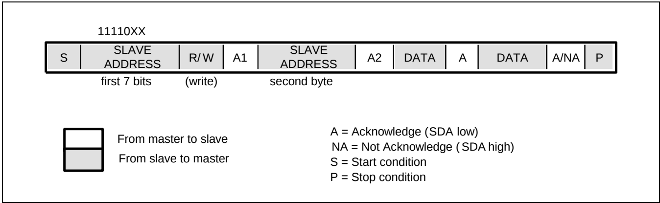
Figure 17-7 主机-发送端用10位地址寻址从机-接收端
