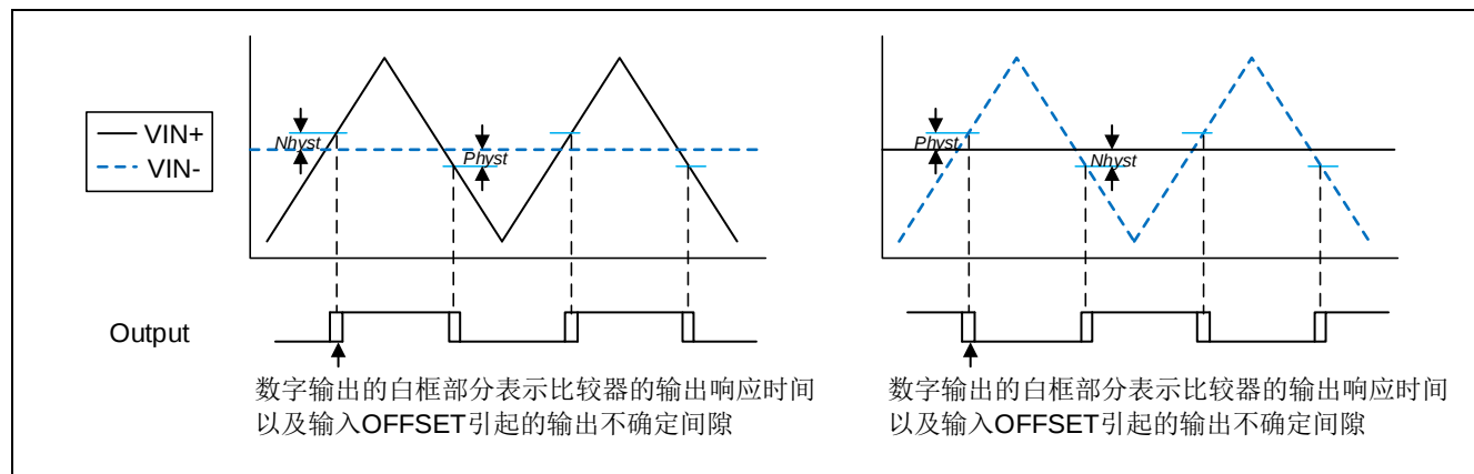
Figure 10-1 单一比较器示意图
