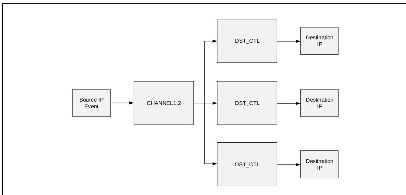
Figure 8-4 单个源触发多个目标
