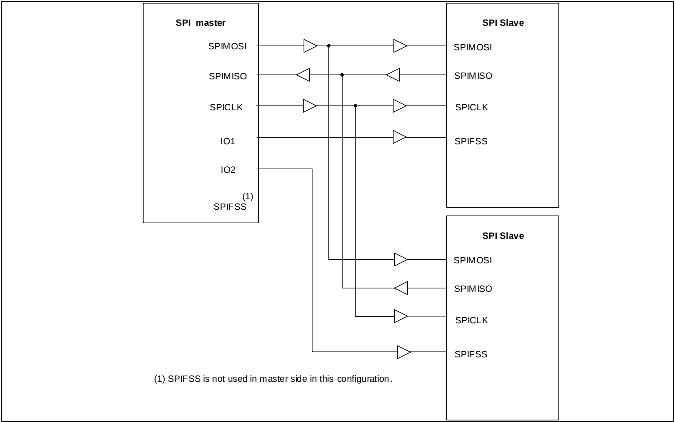
Figure 16-4 SPI 主机连接到两个SPI从机
