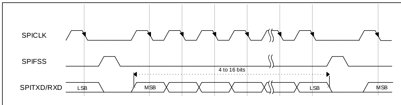
Figure 16-8 Motorola SPI 帧格式（连续传输），SPO = 0 和 SPH = 1
