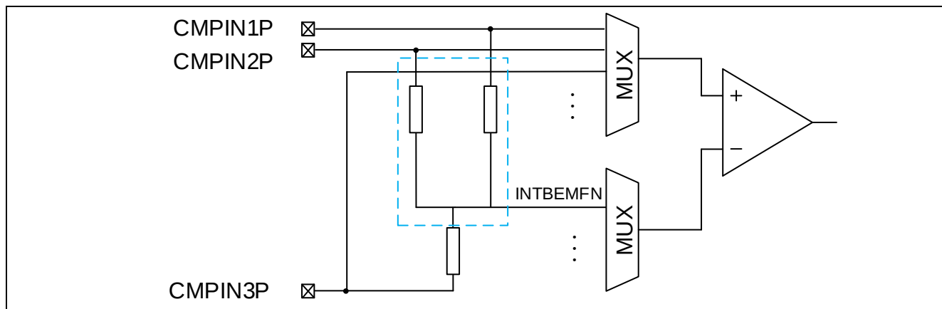
Figure 10-6 反电动势检测功能
