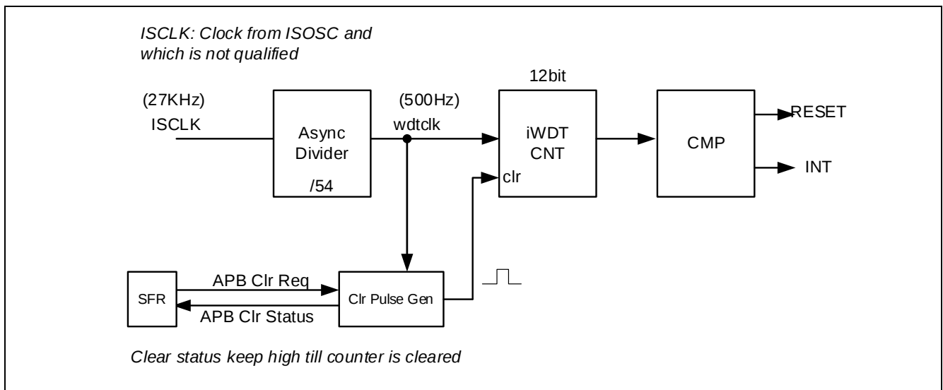
Figure 5-9 IWDT 结构框图
