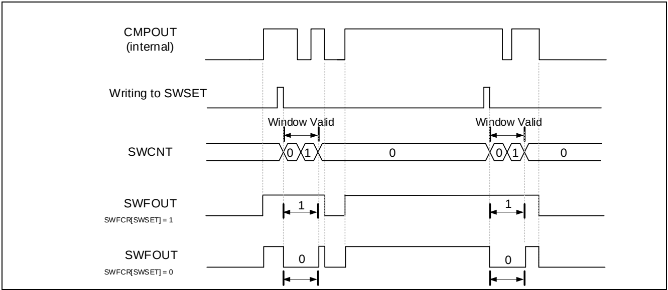
Figure 10-4 SWFCR[SWSET]不同值时，软件窗口滤波机制
