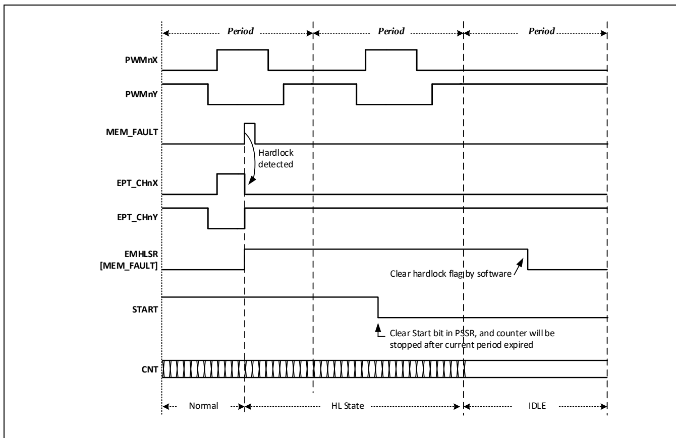
Figure 14-33 硬锁止模式
