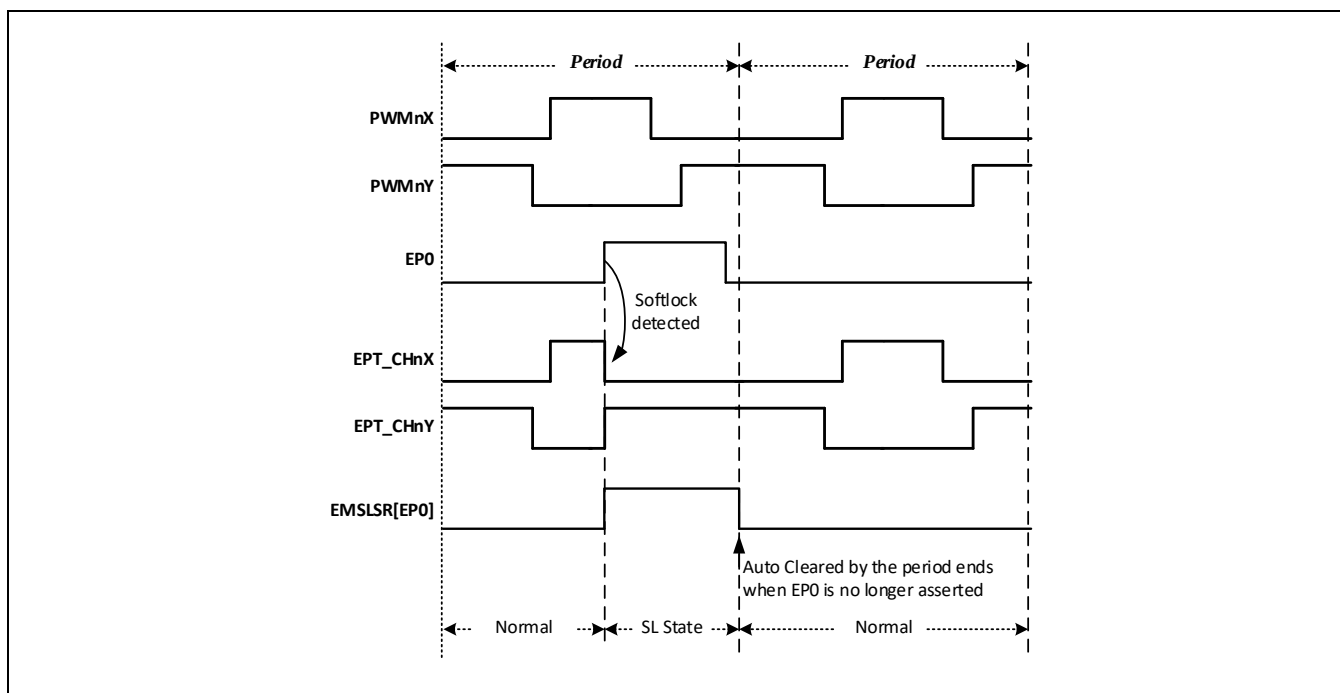
Figure 14-32 软锁止模式
