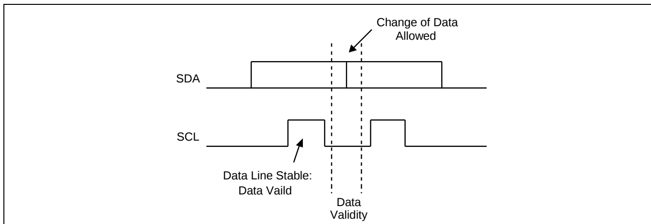
Figure 17-2 数据有效性
