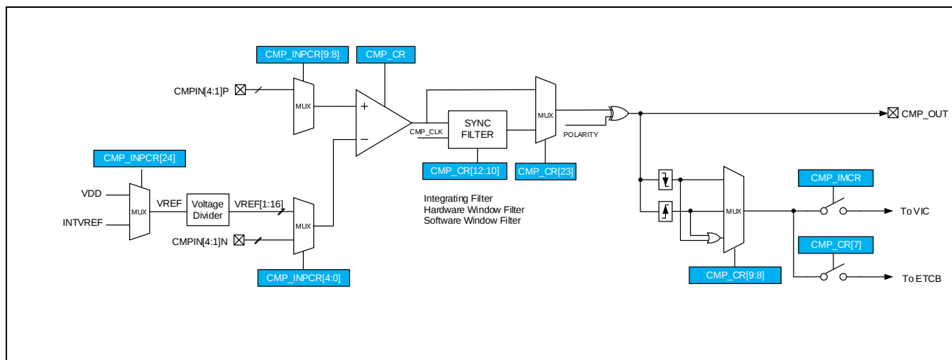
Figure 10-2 比较器结构示意图
