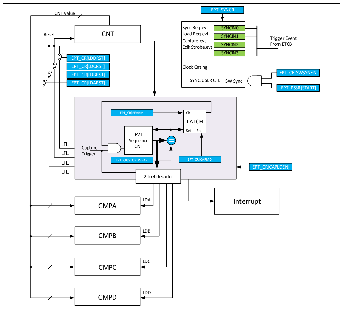
Figure 14-35 捕捉模式结构框图
