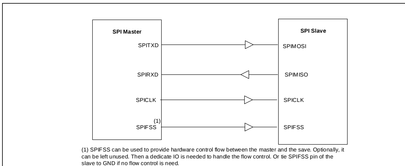
Figure 16-3 SPI主机连接1个SPI从机
