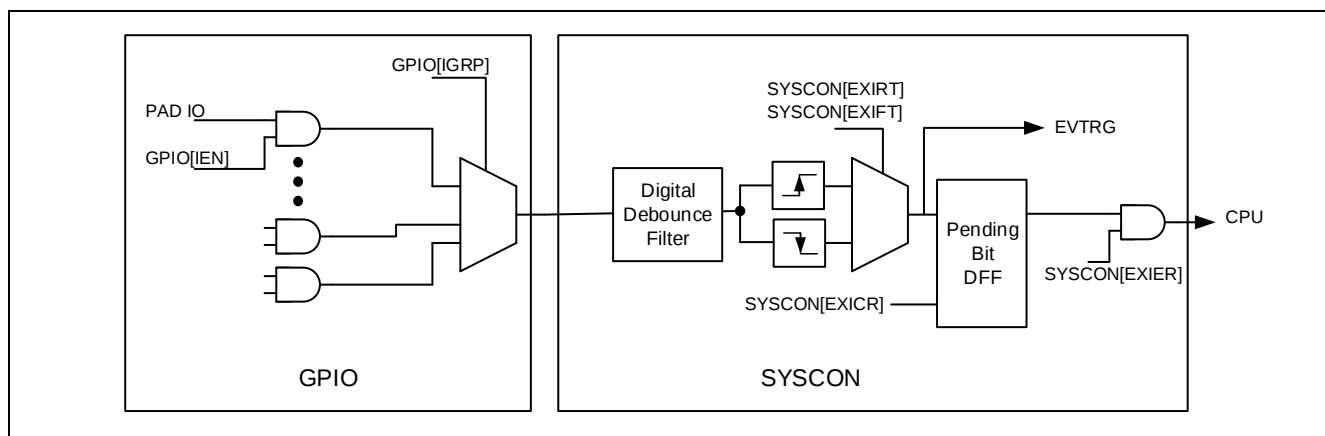
Figure 5-8 外部中断结构示意图
