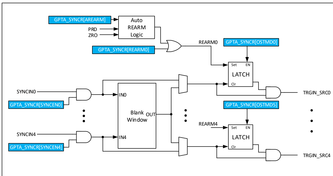
Figure 13-16 同步触发输入
