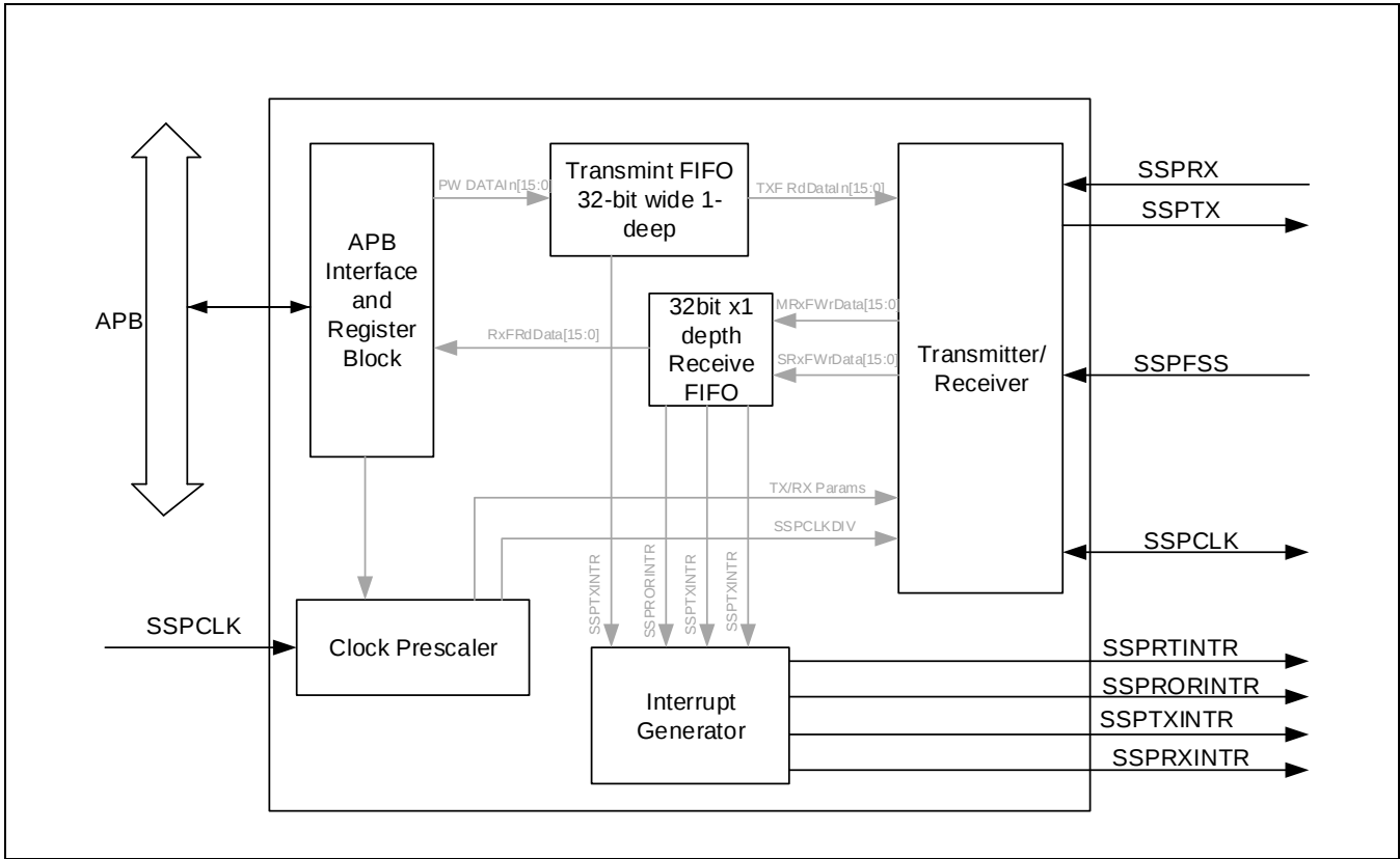
Figure 16-1 SPI 模块框图
