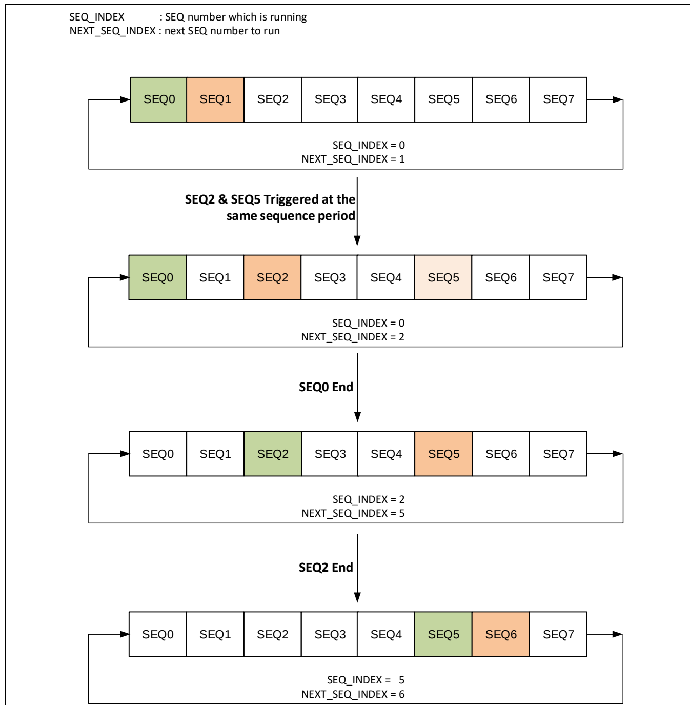
Figure 9-7 同时触发示意图
