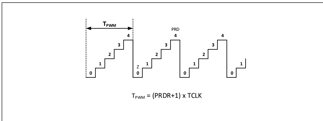
Figure 13-6 计数器工作模式
