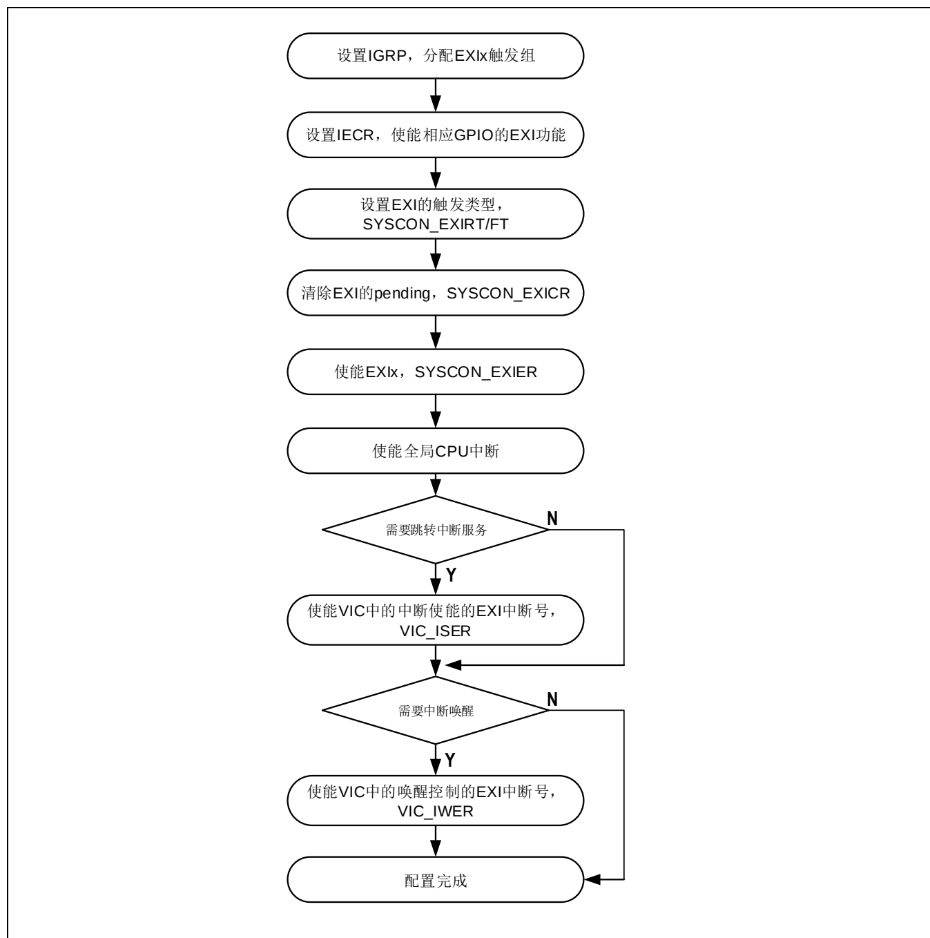
Figure 7-3 GPIO外部中断配置流程
