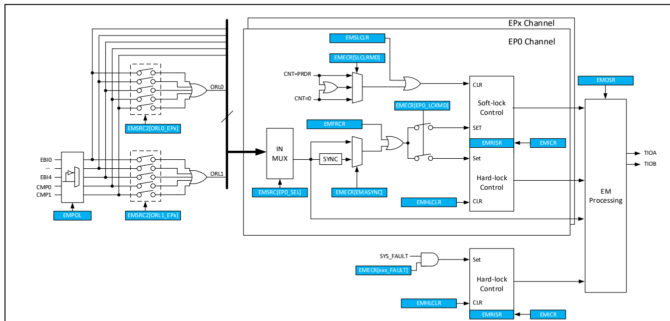
Figure 14-31 紧急模式控制模块
