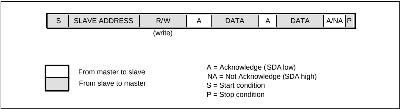
Figure 17-6 主机-发送端寻址从机
