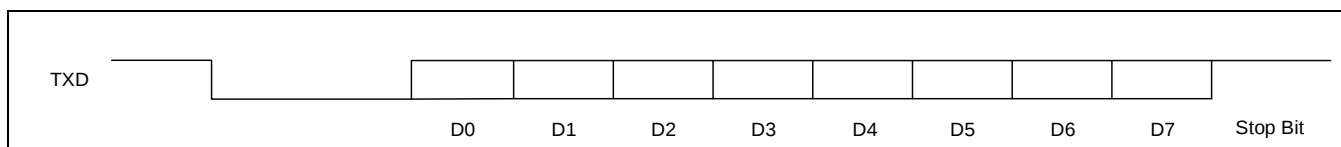
Figure 15-4 数据发送
