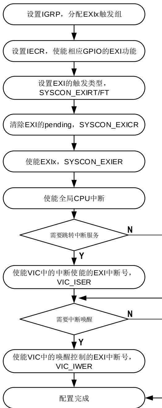
Figure 7-4 GPIO外部中断配置流程
