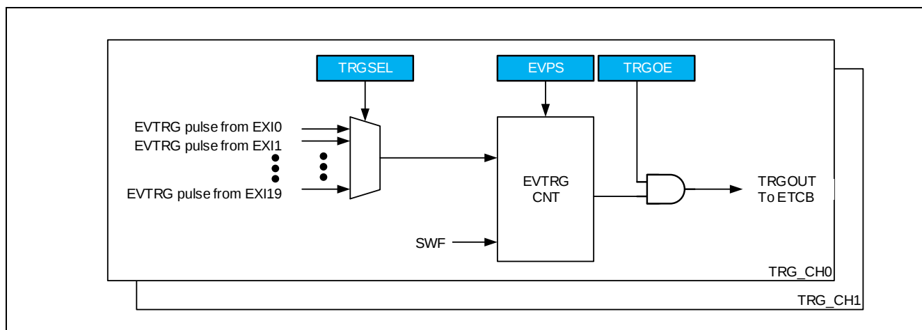
Figure 5-13 SYSCON 外部事件触发控制逻辑
