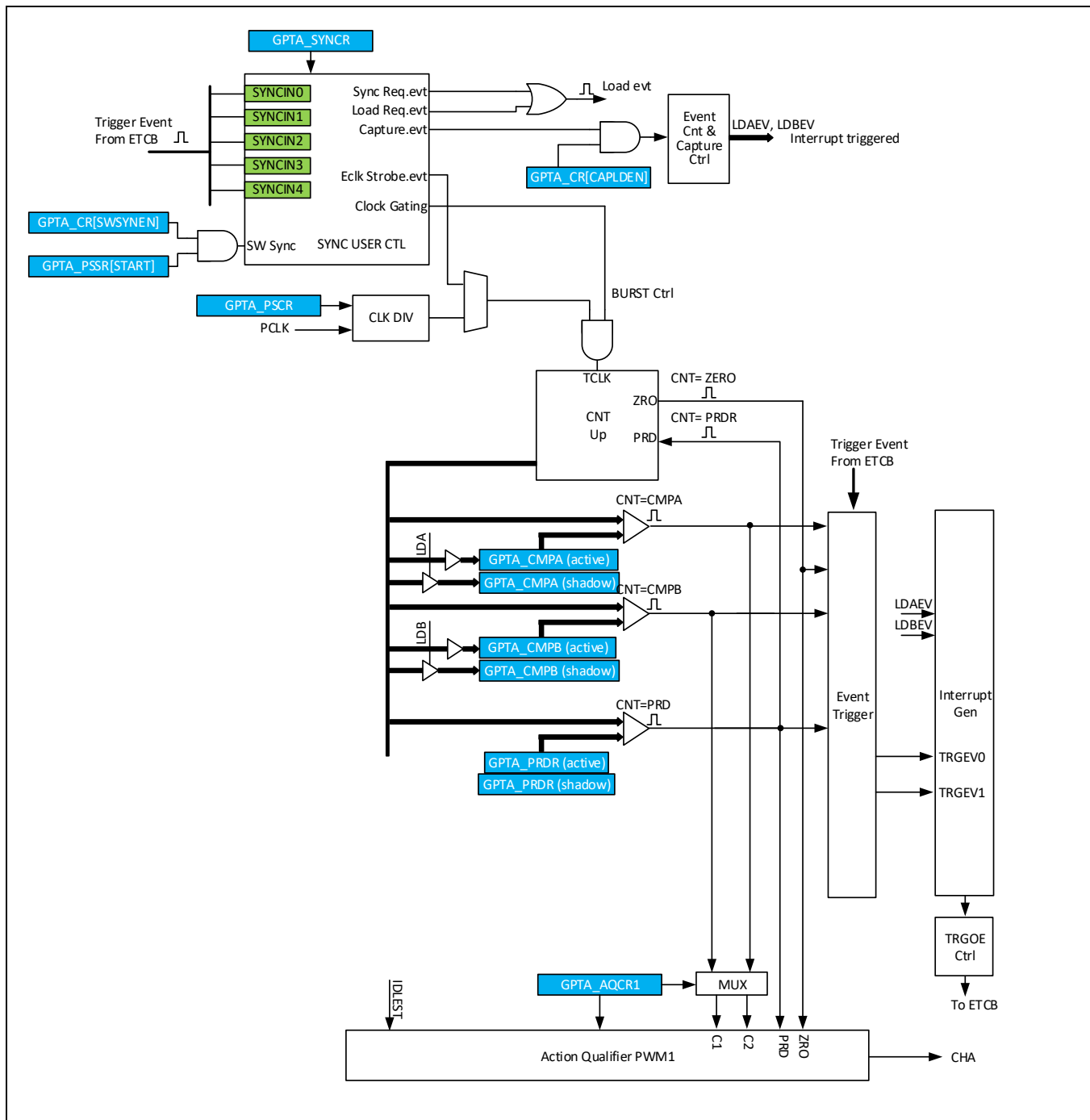
Figure 13-1 模块结构示意图
