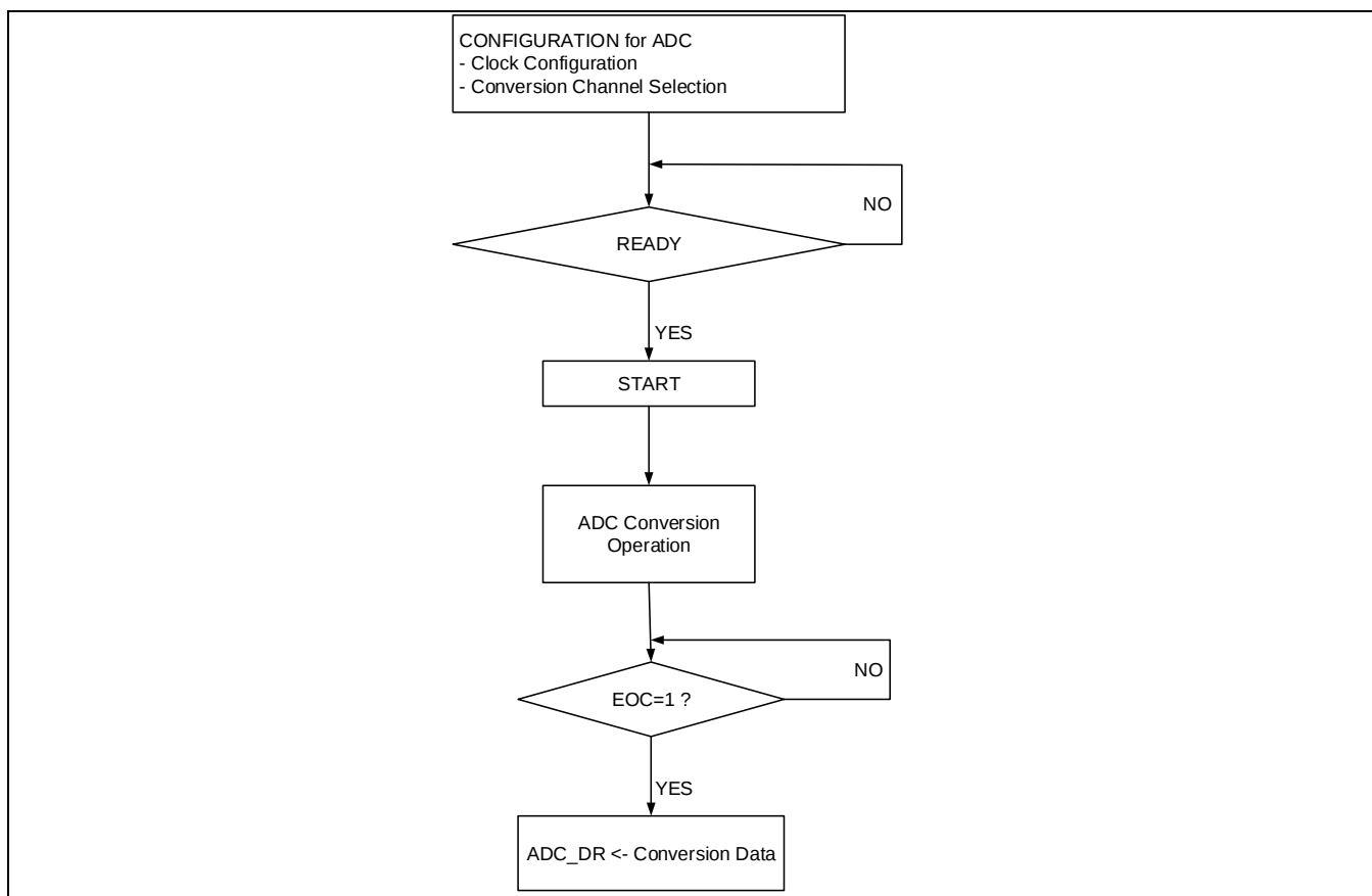
Figure 9-9 ADC工作流程图
