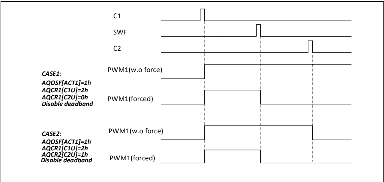
Figure 14-20 一次性软件强制输出
