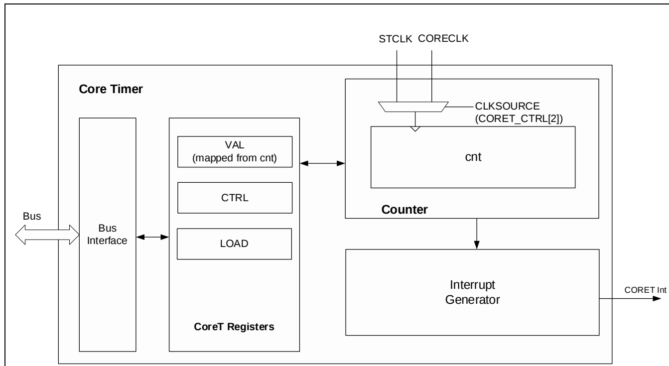
Figure 3-1 CORET模块框图
